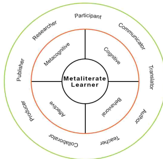
Fig. 3. Metaliteracy
